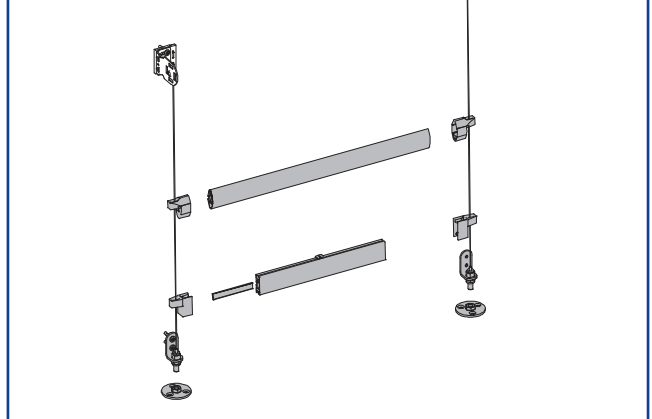
WIRE GUIDE
